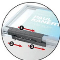
Ausweishalter PUSHBOX TRIO, Schiebemechanismus
